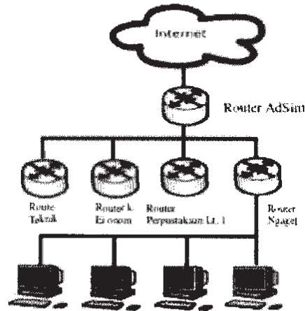
Gambar 2. Topologi Jaringan Internet Kampus
