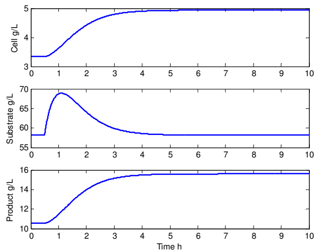
Gambar 4. Profil variabel output ketika terjadi perubahan konsentrasi substrate dari 100 g/L menjadi 120 g/L pada menit ke 30.
