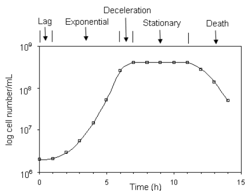
Gambar 1. Kurva pertumbuhan mikroorganisme sistem batch
