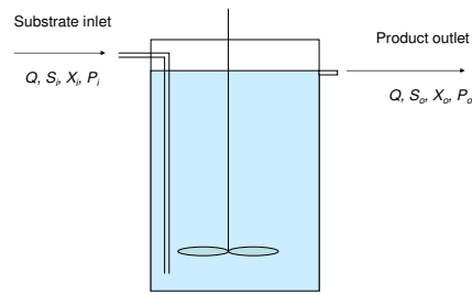
Gambar 2. Sistem fermentasi
