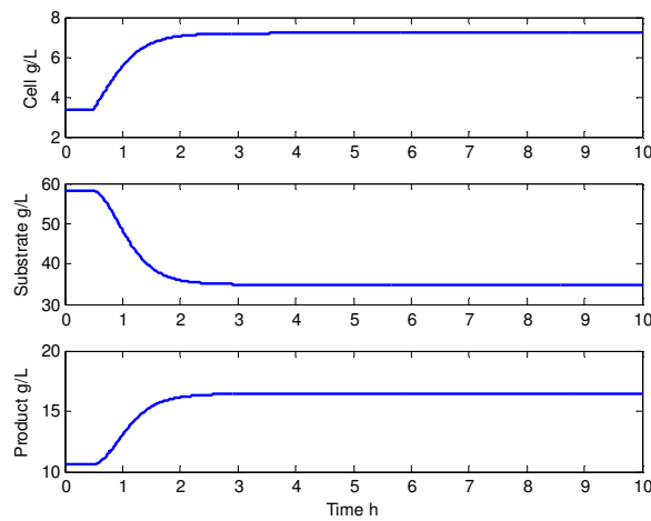
Gambar 6. Profil perubahan variabel output: konsentrasi sel berubah dari 0 g/L menjadi 2 g/L pada menit ke 30
