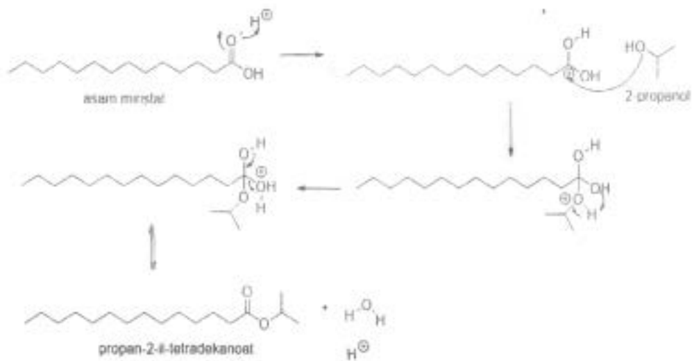
Gambar 2. Mekanisme reaksi sintesis senyawa propan-2-il-tetradekanoat
