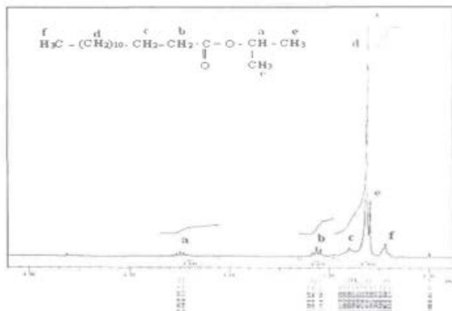
Gambar 4. Spektrum ^1\text{H-NMR} senyawa propan-2-il-tetradekanoat
