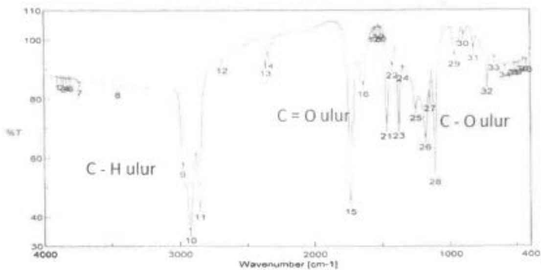
Gambar 3. Spektrum FTIR senyawa propan-2-il-tetradekanoat pada pellet KBr
