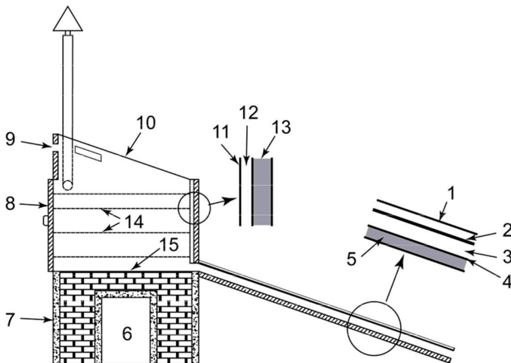
Gambar 3. Penampang melintang tampak samping pengering: 1. penutup transparan (kaca); 2. lempeng penyerap panas; 3. spasi ruang masuk udara; 4. lapisan bawah spasi ruang gerak udara; 5. insulasi; 6. tungku pembakaran biomassa; 7. media penyimpan panas; 8. pintu rak pengering; 9. ventilasi; 10. atap transparan; 11. dinding internal rak; 12. spasi kosong tempat aliran asap; 13. dinding luar rak dengan insulasi; 14. rak/tray pengering; 15. plat bawah rak/tray
