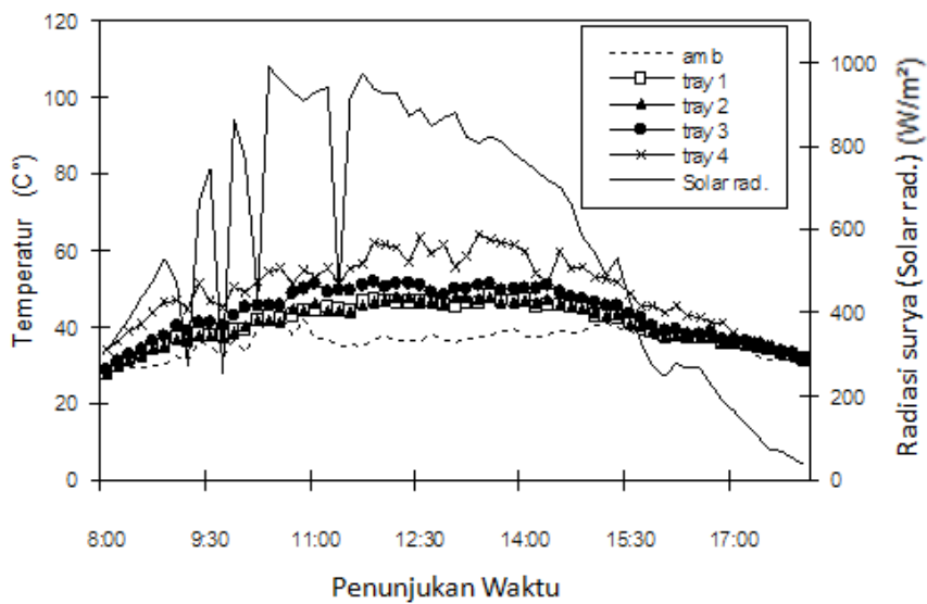
Gambar 5. Temperatur dalam rak/tray pengering dengan pengoperasian dengan tenaga surya
