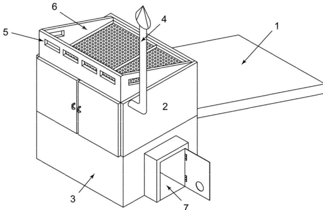
Gambar 2. Pengering tenaga surya dengan sistem bekap biomassa. Bagian-bagian sistem: 1. kolektor surya, 2. kotak dan rak, 3. media penyimpan panas, 4. cerobong asap, 5. ventilasi, 6. atap transparan, 7. tungku pembakaran biomassa
