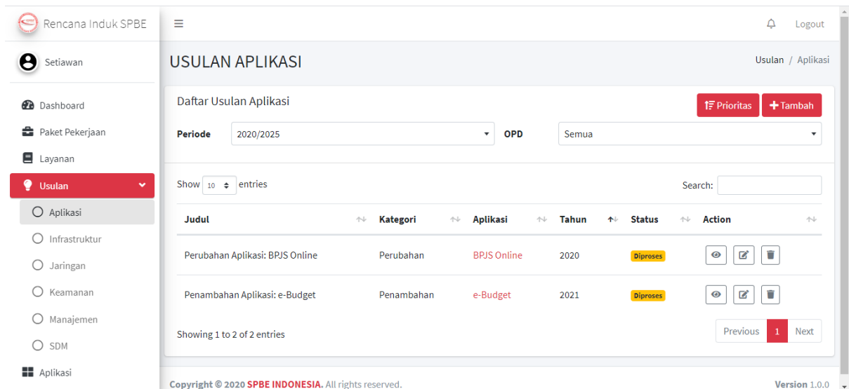
Gambar 66 Tampilan Daftar Usulan Aplikasi untuk Tim
