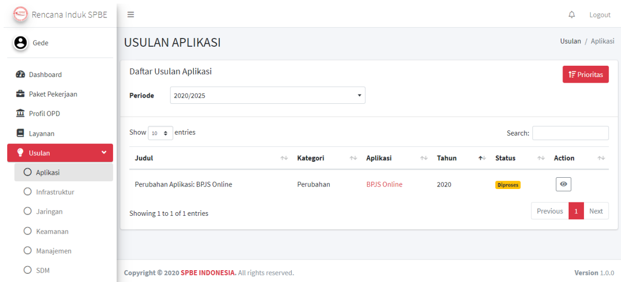
Gambar 65 Tampilan Daftar Usulan Aplikasi untuk OPD dan Admin
