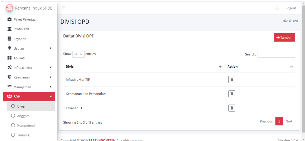
Gambar 52 Tampilan Daftar Divisi OPD
