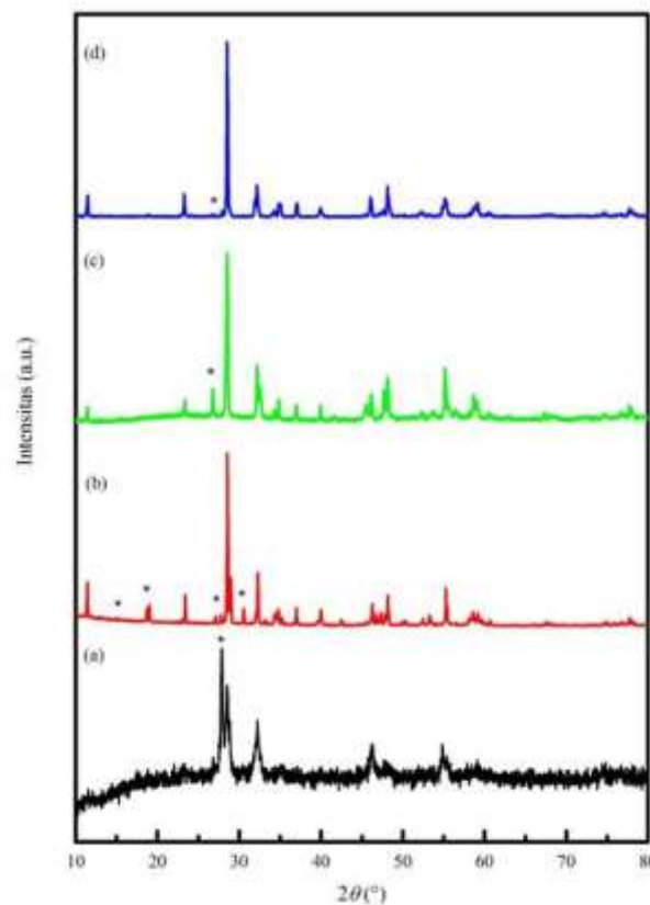
Gambar 2 Pola difraksi oksida hasil sintesis dengan menggunakan metode sol gel pada berbagai kondisi yang dibakar pada suhu 800^\circ\text{C} , (a) perbandingan pengkhelat asam sitrat dan jumlah total mol kation logam yang digunakan adalah 1:1 serta pH 7 , (b) perbandingan pengkhelat asam sitrat dan jumlah total mol kation logam yang digunakan adalah 1:1 serta pH 1-3 , (c) perbandingan pengkhelat asam sitrat dan EDTA, (d) perbandingan pengkhelat asam sitrat dan etilen glikol serta jumlah total mol kation sebesar 1:1:1 pada kondisi pH asam. Tanda * menunjukkan beberapa puncak selain fasa BIMEVOX.
