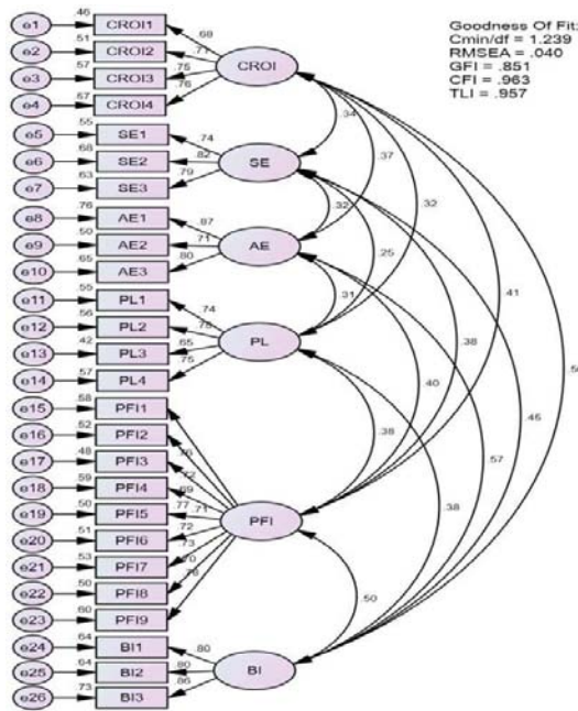
Gambar 1 Model Pengukuran
