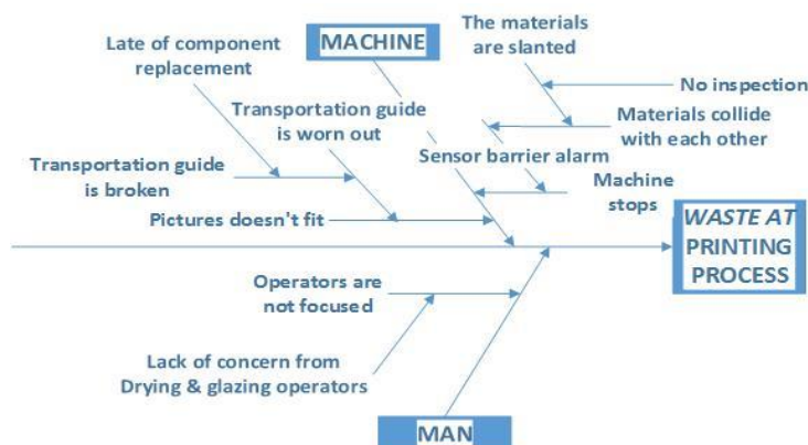
Gambar 6. Akar penyebab masalah pada proses printing
