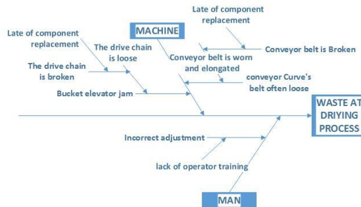
Gambar 5. Akar penyebab masalah pada proses drying
