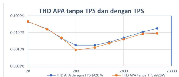
Gambar 10. Grafik THD APA tanpa TPS dan dengan TPS
