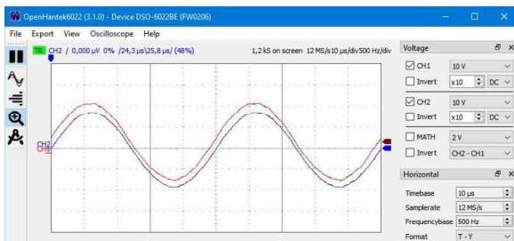
Gambar6. Bentuk gelombang tegangan output APA dan TPS sisi positif.
