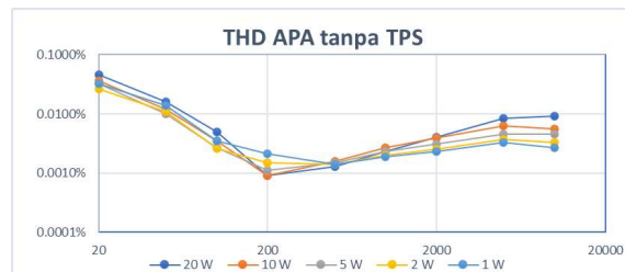
Gambar8. Grafik THD APA tanpa TPS.
