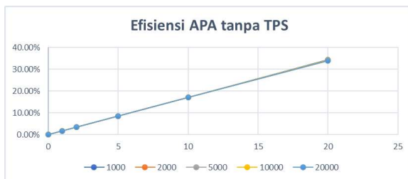
Gambar 11. Grafik Efisiensi APA tanpa TPS
