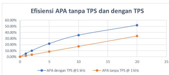
Gambar 13. Grafik Efisiensi APA tanpa TPS dan dengan TPS
