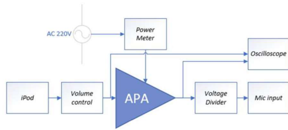
Gambar 7. Konfigurasi alat ukur untuk mengukur THD dan efisiensi.
