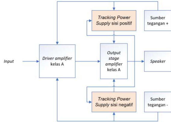
Gambar 1. Diagram blok sistem APA dengan TPS.
