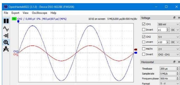
Gambar 3. Bentuk gelombang tegangan input dan output APA
