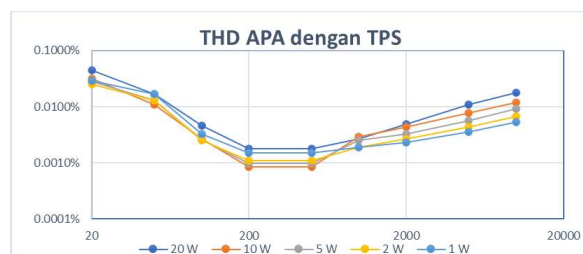
Gambar9. Grafik THD APA dengan TPS.
