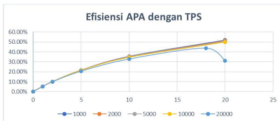
Gambar 12. Grafik Efisiensi APA dengan TPS
