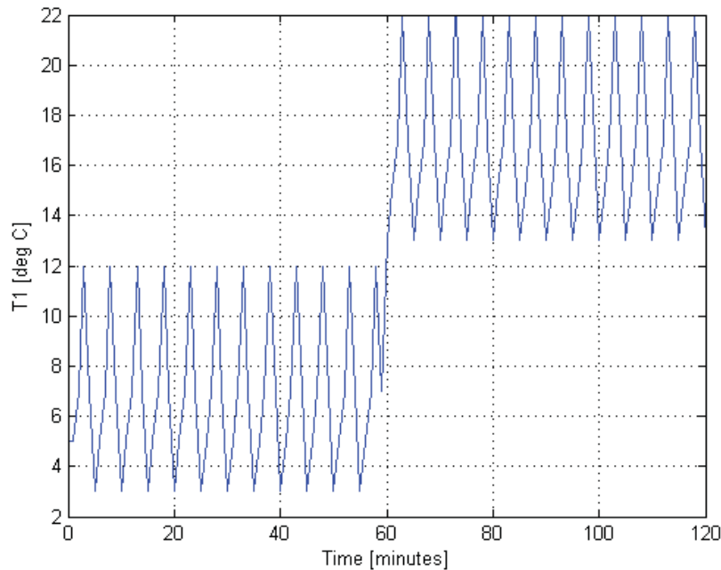
Fig. 3. Input profile.
