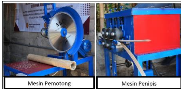
Gambar 5. Peningkatan Aset melalui Pemberian Mesin Potong dan Mesin Penipis Bambu
