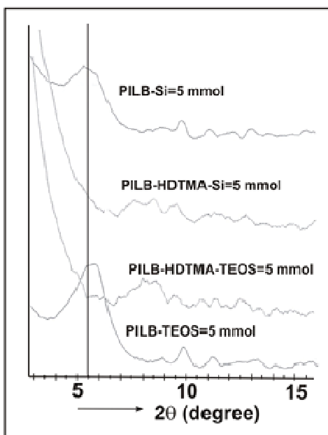
Gambar 3. Difraktogram XRD bentonit terpillar secara langsung oleh Si (PILB-Si), TEOS (PILB-TEOS), dan secara tidak langsung (PILB-HDTMA-Si dan PILB-HDTMA-TEOS)
