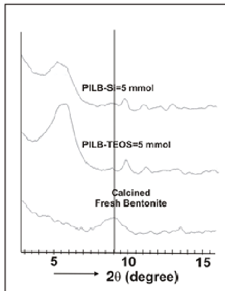
Gambar 2. Difraktogram XRD bentonit terpillar
