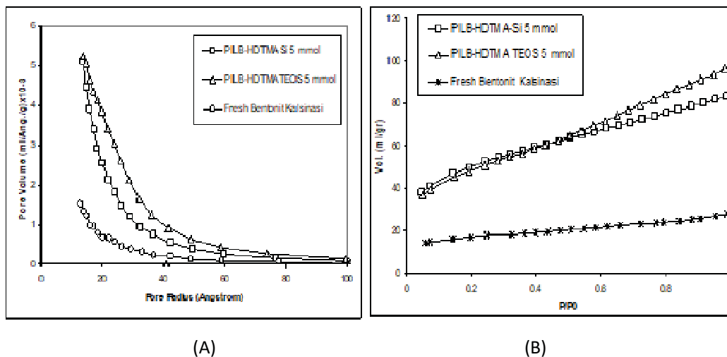
Gambar 4. (A) Kurva distribusi ukuran pori, (B) Kurva adsorpsi gas N_2 bentonit alam ( fresh bentonite ), bentonit terpillar Si secara tidak langsung (PILB-HDTMA-Si), bentonit terpillar TEOS secara tidak langsung (PILB-HDTMA-TEOS)
