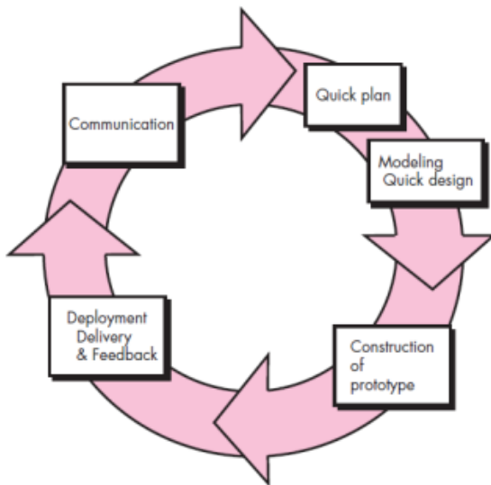
Gambar 1. Metode Prototipe
