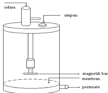
Gambar 3. Alat penguji membran (Dead End)
