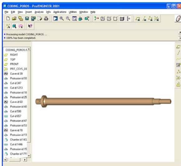
Gambar 6. Pemodelan 3D Poros
