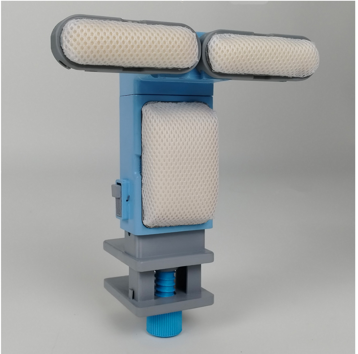
Gambar 1 - Tampak Perspektif
